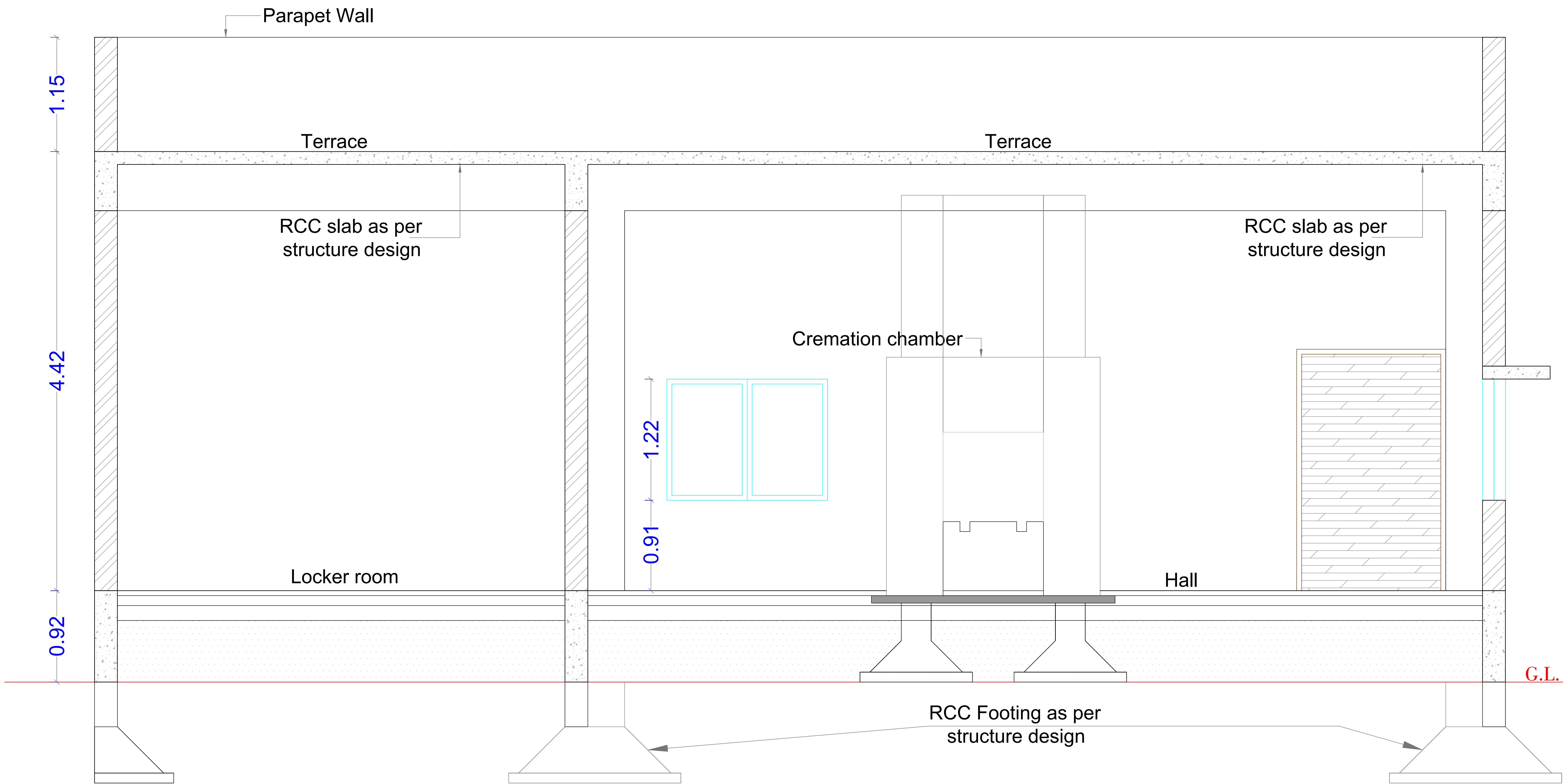
SECTION A-A'
