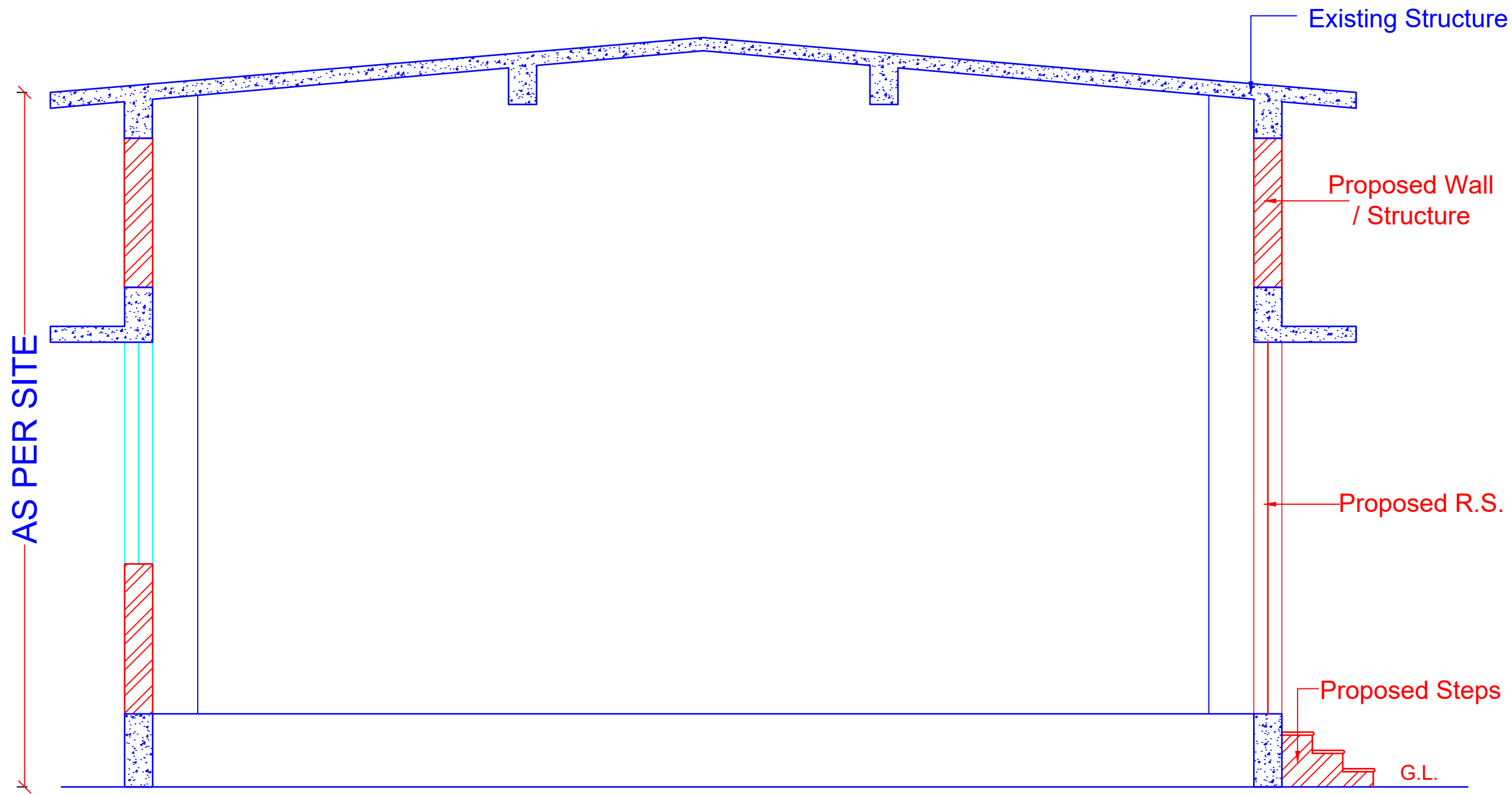
SECTION A-A'
