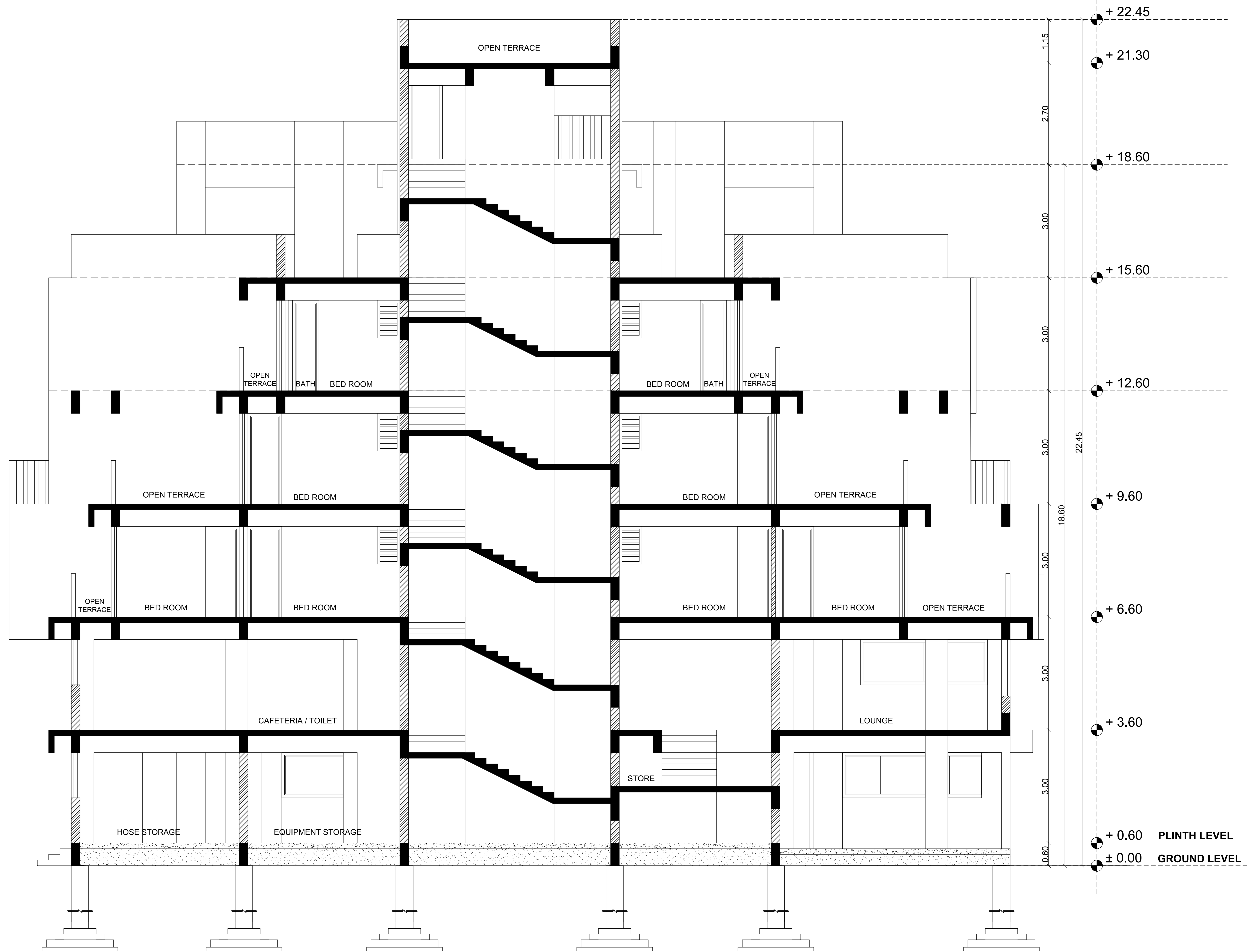
SECTION- A-A"
